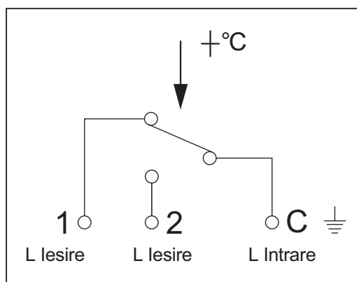
Schema cablare
